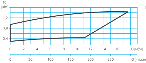
RV2-F 65-120
