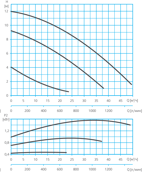
RA2-F 65-120 (3~400 V)
