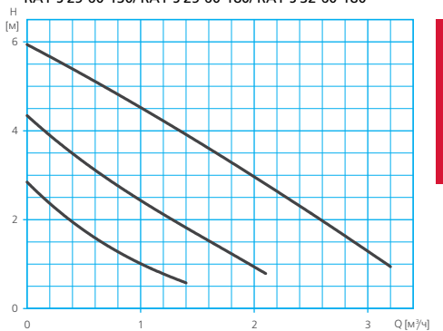
RA1-S 15-60-130/ RA1-S 20-60-130/ RA1-S 20-60-180/ RA1-S 25-60-130/ RA1-S 25-60-180/ RA1-S 32-60-180
