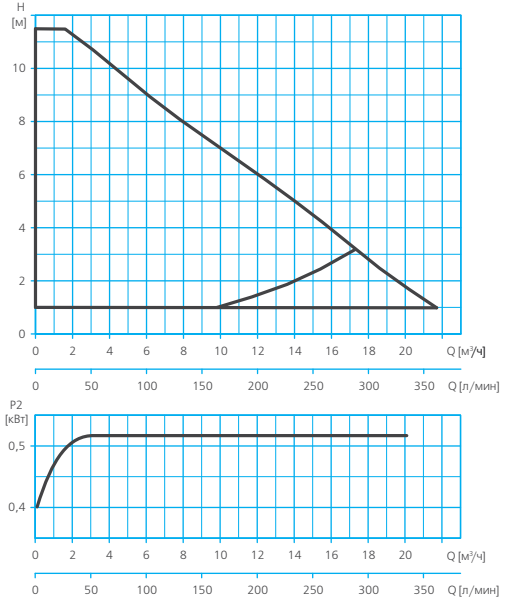
NMT F 40
