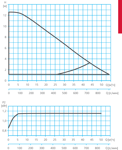
NMT F 65
