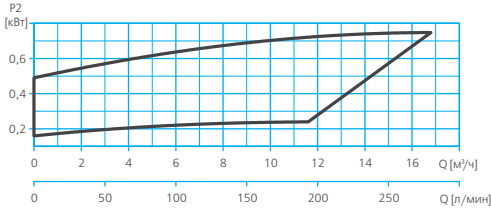
RE1-F 50-100
