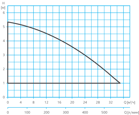
RE2-F 65-60
