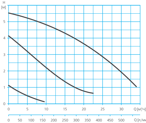
RA1-F 65-70 (3~400 V)
