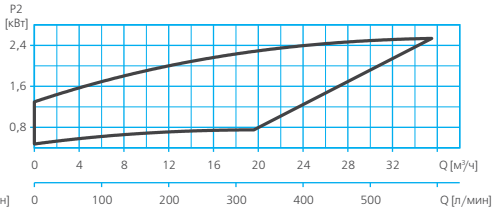
RV2-F 80-120
