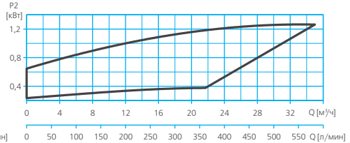
RV1-F 80-120
