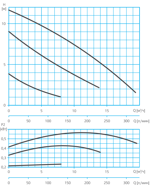
RSAN-F 40-120
