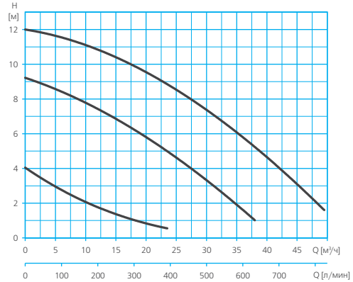
RA1-F 65-120 (3~400 V)
