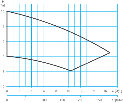
RE1-F 40-100
