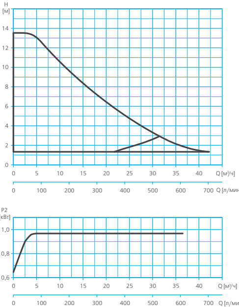
NMT F 50
