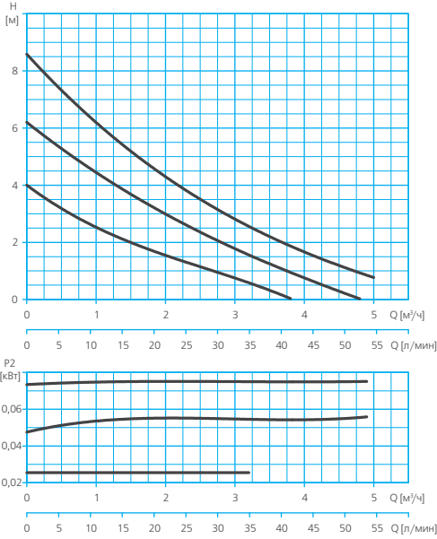
NMT 25/80 – 180/ NMT 32/80 – 180
